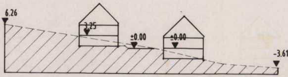
GELÄNDESNITT M.: 1:500
