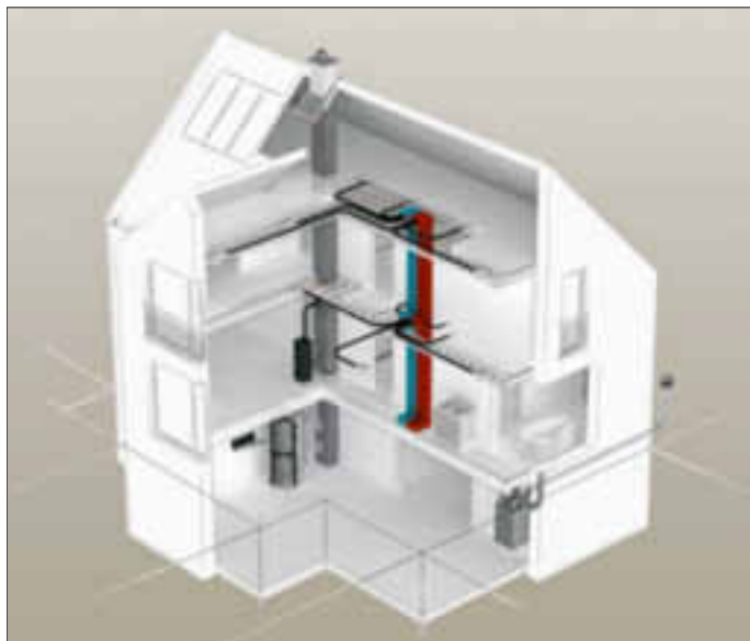
Raffinierte Konstruktion: Ein Lüftungsnetzwerk sorgt für frische Luft in den eigenen vier Wänden, ohne dass im Winter wertvolle Heizwärme verloren geht. Grafik: Erlus/interPress
